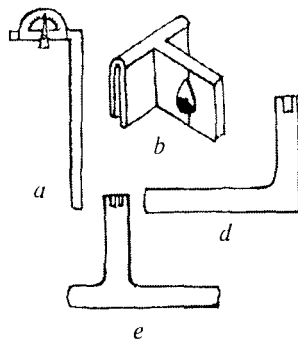
44-rasm. Proyeksion o'lchamlarni o'lchaydigan chizg'ichlar: a — goniometrli chizg'ich; b , d — bel chuqurliklarini o'lchash uchun chiz- g'ichlar, e — kurak botiqligini o'lchash uchun chizg'ich.
